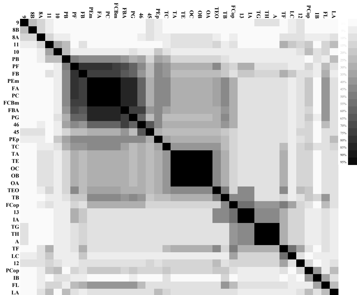
Abb. 8: OSA-Clusterplot für die gewichteten Daten unter der AVERAGE Parameterkonstellation. Siehe Legende zu Abb. 3 für die Interpretation der Darstellung.
