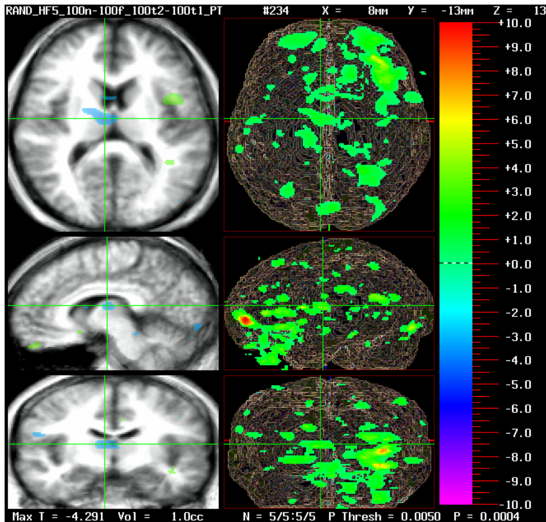
Abb. 13: Ergebnisse der DS-Analyse für das linke Zerebellum, projiziert auf das gemittelte strukturelle T1-Bild aller Probanden. Das Fadenkreuz zeigt einen Cluster mit 487 signifikanten Voxeln im rechten mediodorsalen Thalamus. Sonstige Konventionen entsprechen denen von Abb. 12.
