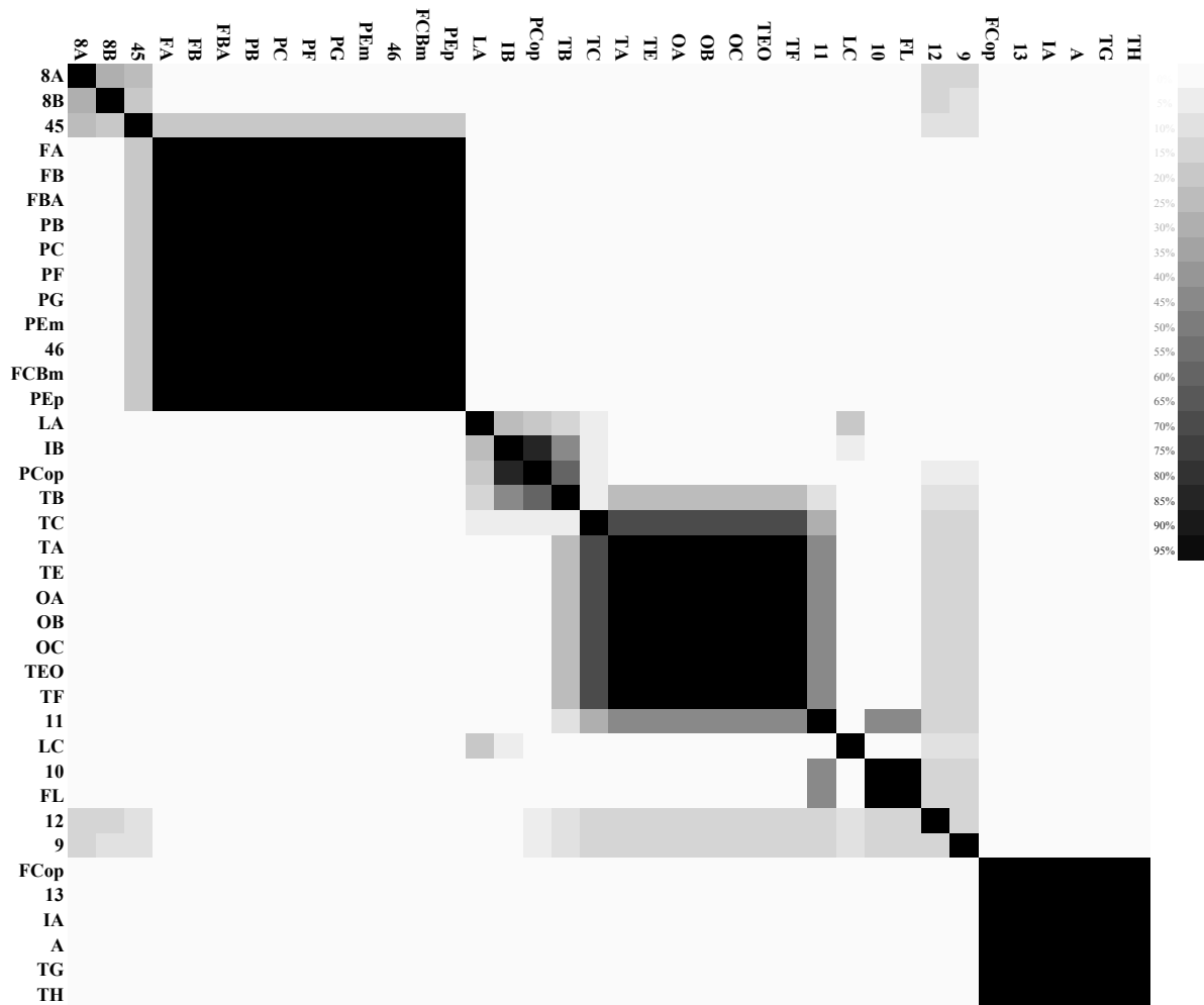
Abb. 3: OSA-Ergebnisse für die gewichteten Daten unter der BALANCE-Bedingung. Die grauwert-kodierten Einträge der Matrix geben die Assoziation aller Paare von Arealen an (d. h. die Häufigkeit, mit der zwei Areale über alle OSA-Zyklen hinweg dem gleichen Cluster zugeordnet wurden) – siehe Grauwertskala am rechten Bildrand. Die Areale wurden so sortiert, dass gemeinsame Clusterzugehörigkeiten optimal visualisiert werden.
