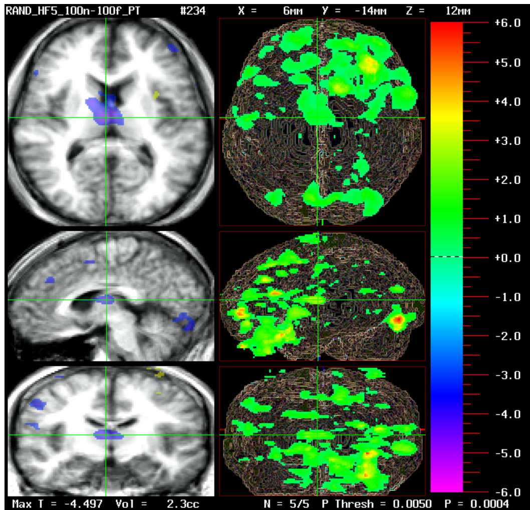
Abb. 12: Ergebnisse der ON-OFF-Analyse für das linke Zerebellum, projiziert auf das gemittelte strukturelle T1-Bild der Patienten. Alle signifikanten Voxel ( p < 0,005 , unkorrigiert für multiple Vergleiche) sind als farbkodierte t-Wert-Karte dargestellt, unabhängig von der Grösse des zugehörigen Clusters. Die Darstellung des Hirns entspricht der radiologischen Konvention. Linke Spalte: Das Fadenkreuz zeigt einen Cluster mit 1.074 signifikanten Voxeln mit Schwerpunkt im rechten mediodorsalen Thalamus. Rechte Spalte: Darstellung als "birdcage image", in dem die absoluten t-Werte aller Voxel auf die drei Hauptebenen projiziert werden (analog zu den "glass brains" des Softwarepakets SPM99).
