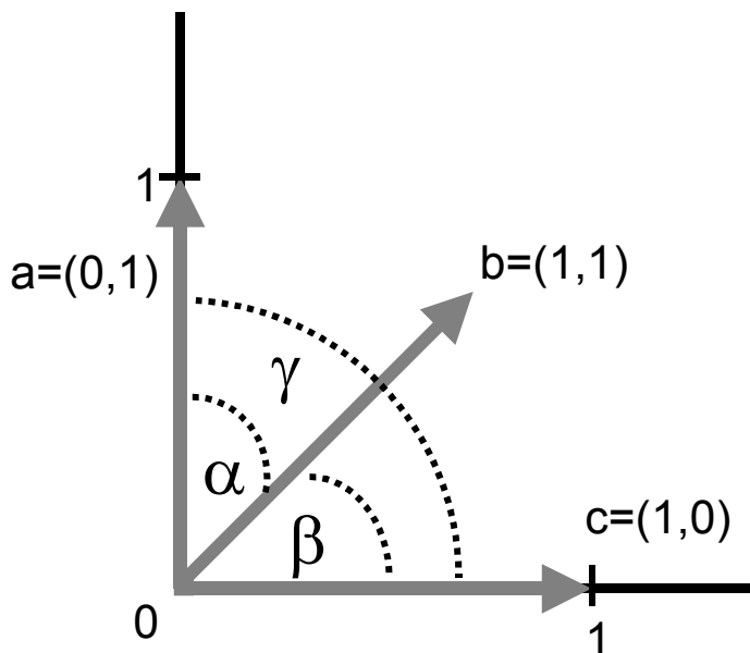
Abb. 11: Drei hypothetische Messreihen mit jeweils zwei Messungen, dargestellt als Vektoren a, b und c.
