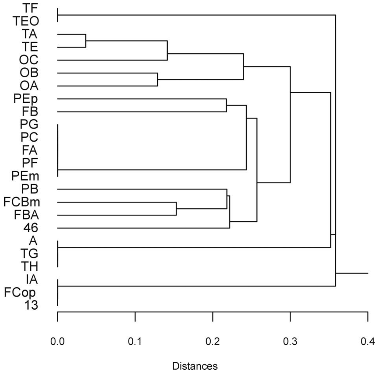
Abb. 5: Hierarchische Baumdarstellung der OSA-Ergebnisse für die gewichteten Daten unter der HIGH REPULSION Parameterkonstellation. Die Analyse wurde auf die Areale der aus allen Analysen hervorgehenden drei Hauptcluster beschränkt (vgl. Abb. 9). Von links nach rechts ist die Verschmelzung der Areale zu hierarchisch angeordneten Clustern dargestellt. Initial wird jedes Areal als ein separater Cluster aufgefasst (Distanz = 0). In jedem Verschmelzungsschritt werden dann die zwei ähnlichsten Areale zu einem Cluster zusammengefasst. Die Verschmelzung wird solange fortgesetzt, bis alle Areale in einem Cluster liegen. Die Verschmelzungsdistanz wird als der Abstand zwischen den beiden ähnlichsten Arealen zweier Cluster definiert (single linkage). Da die Analyse auf den OSA-Resultaten, nicht auf den originalen neuronographischen Daten, aufsetzt, zeigt die Skala die Euklidischen Distanzen zwischen den Assoziationsvektoren einzelner Areale bzw. Clustern von Arealen. Umgekehrt lässt sich der Graph von rechts nach links lesen und dann als Prozess der Aufspaltung des Netzwerks in segregierte Cluster bzw. Areale interpretieren. Bei dieser Lesart ist erkennbar, dass bei HIGH REPULSION die Aufspaltung des Netzwerks schon früh (bei einer Distanz von ca. 0,35) erfolgt. Bereits ab einer Distanz von 0,2 erfolgt dann kaum noch eine weitere Differenzierung der Clusterstruktur.
