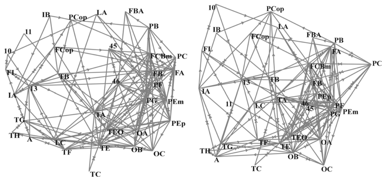
Abb. 10: Zwei repräsentative Beispiele der NMDS-Analysen, die auf den gewichteten neuronographischen Daten ausgeführt wurden. Der Abstand zweier Areale in diesen Plots ist ein inverses Maß für die Ähnlichkeit ihrer Interaktionsmuster. Für den linken Plot wurde das STRESS-Gütekriterium (FIT=1, gebunden) zur Optimierung des Modellfits benutzt, für den rechten Plot das SSTRESS-Gütekriterium (FIT=2, gebunden) (siehe Young et al. 1995 für methodische Details von NMDS). Es ist leicht zu sehen, dass die Parametervariation keinen wesentlichen Einfluss auf die resultierende Clusterstruktur hat.
