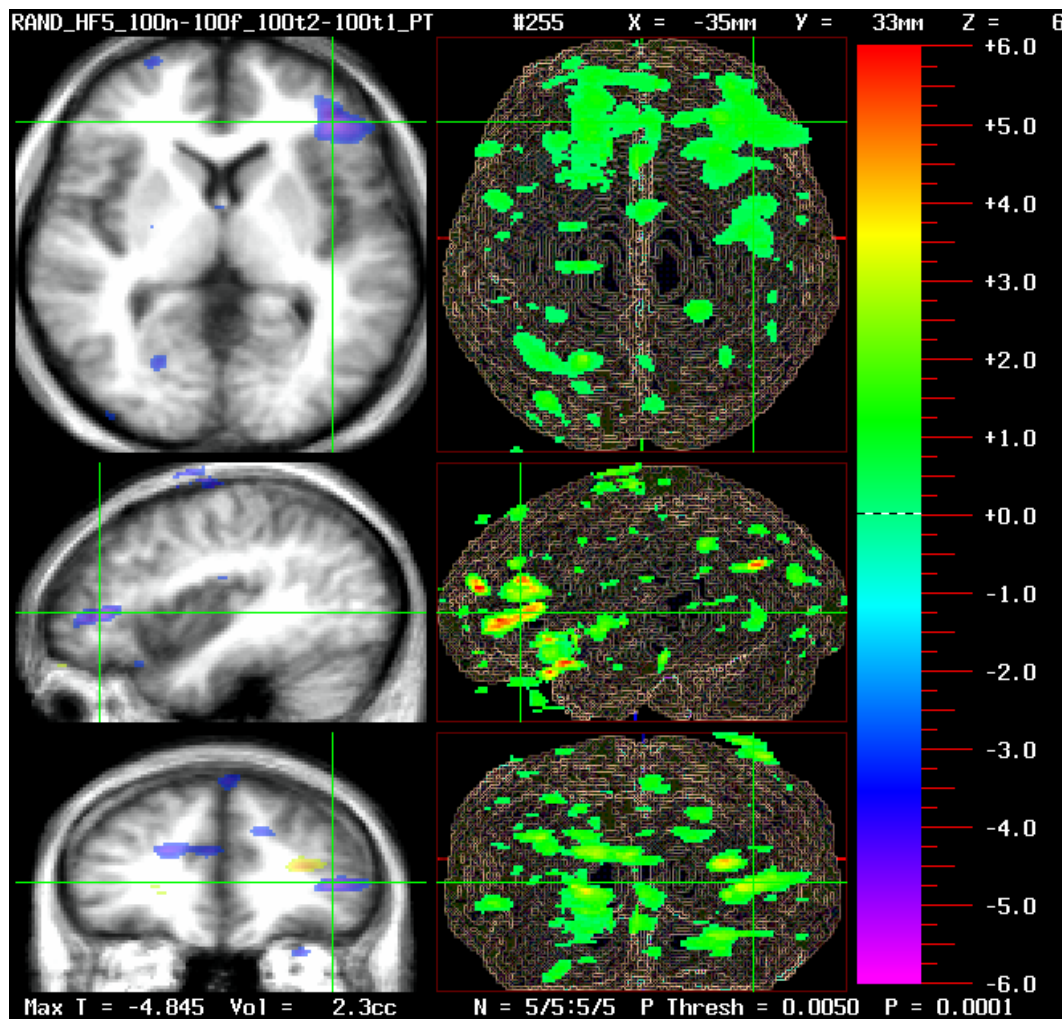
Abb. 14: Ergebnisse der DS-Analyse für das rechte Zerebellum, projiziert auf das gemittelte strukturelle T1-Bild aller Probanden. Das Fadenkreuz zeigt einen präfrontalen Cluster mit 1.054 signifikanten Voxeln im linken lateralen präfrontalen Kortex. Sonstige Konventionen entsprechen denen von Abb. 12.
